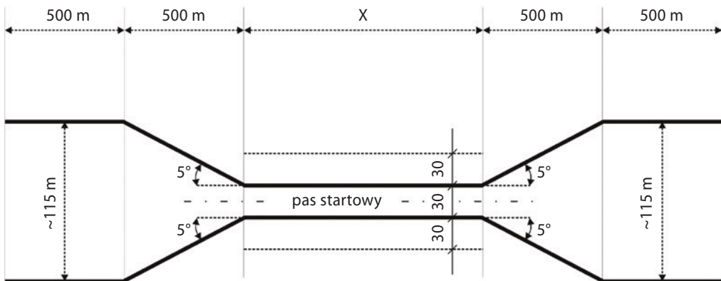
Rycina 1. Rzut poziomy pasa startowego
